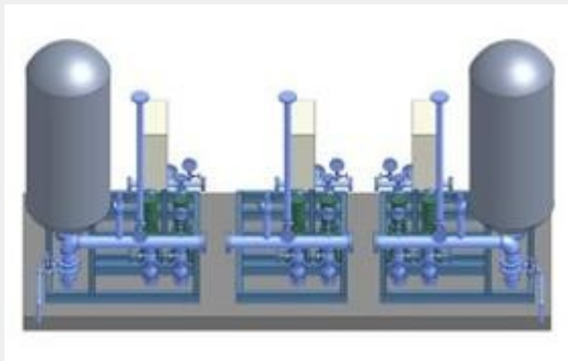
二次侧自动补液稳压建模
