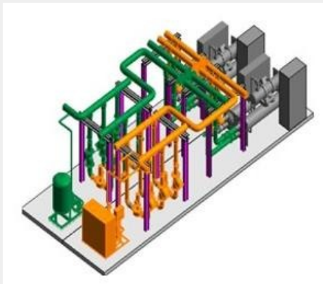
二次侧管路系统
