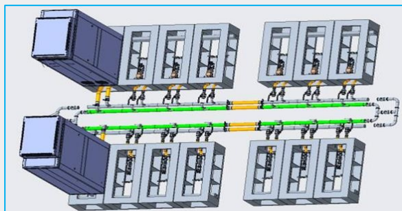
液冷全系统建模
