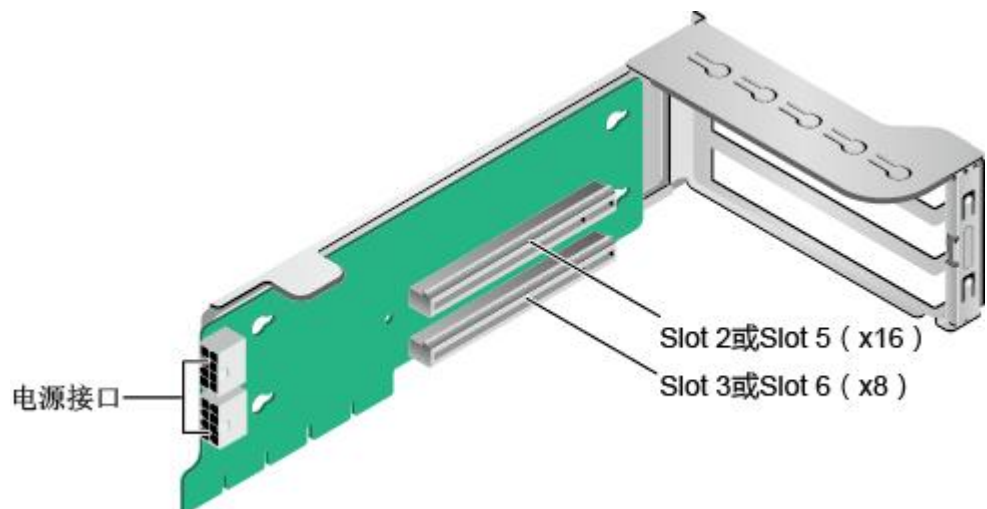
图 3-29 1x8+1x16 Riser 卡 2
