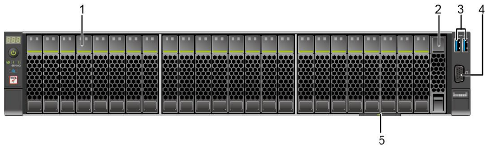
图 3-5 24x2.5 SAS/SATA 硬盘直通配置前面板组件
