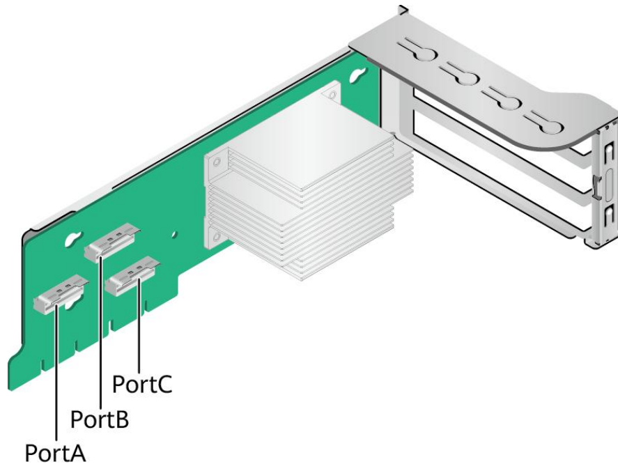
图 3-30 12NVMe 专用 Riser 卡 3
