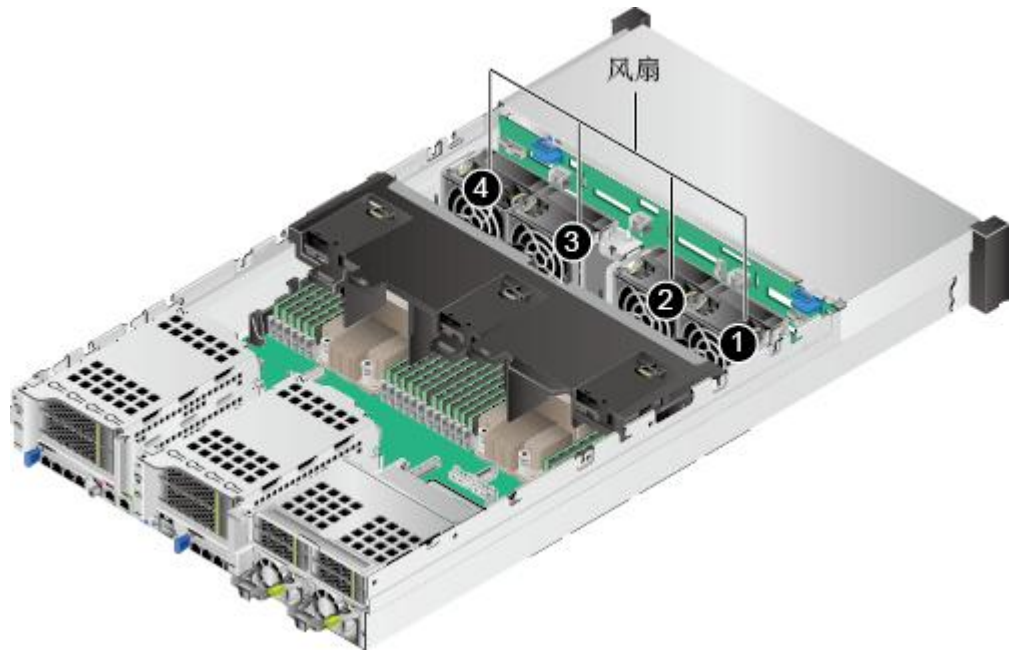
图 3-36 风扇位置图
