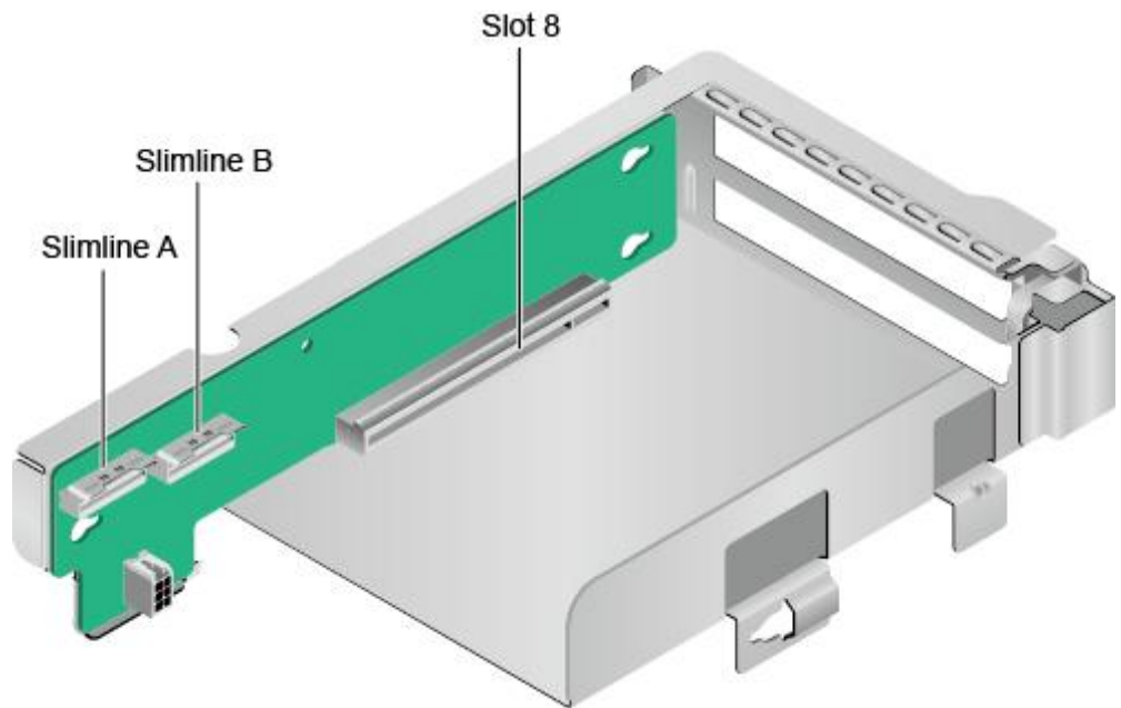
图 3-34 1x16 Riser 卡 7
