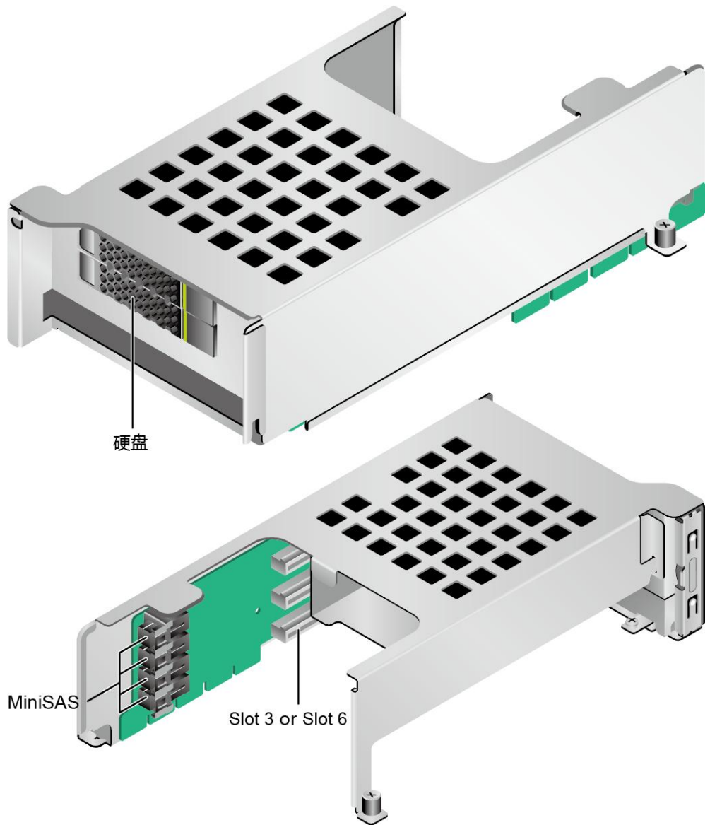
图 3-32 SAS Riser 卡 5
