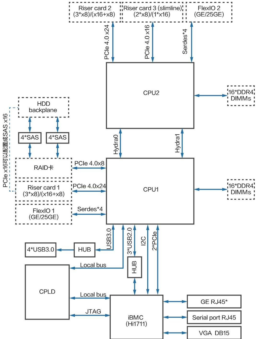
图 2-3 服务器逻辑结构
