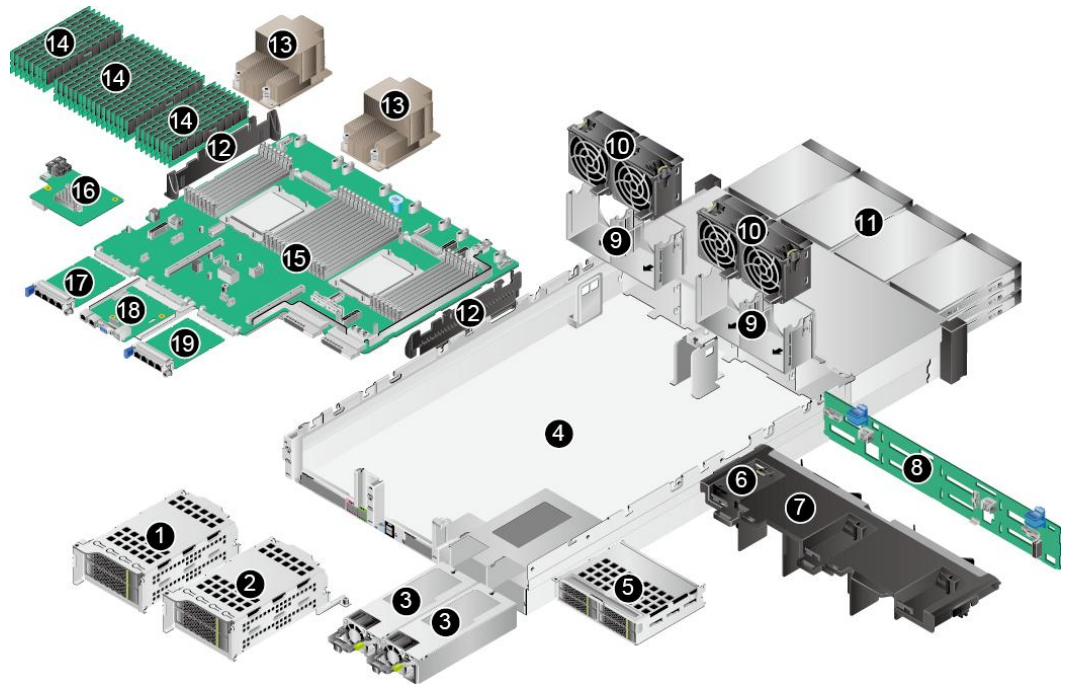
图 2-2 部件
