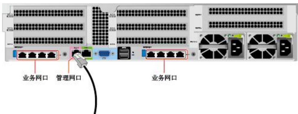
图 6-11 连接网线
