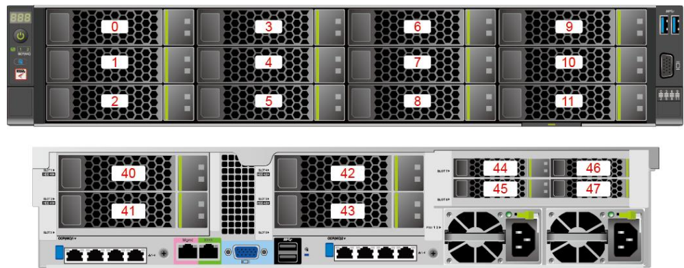
图 3-17 12x3.5 英寸硬盘 EXP 配置硬盘编号
