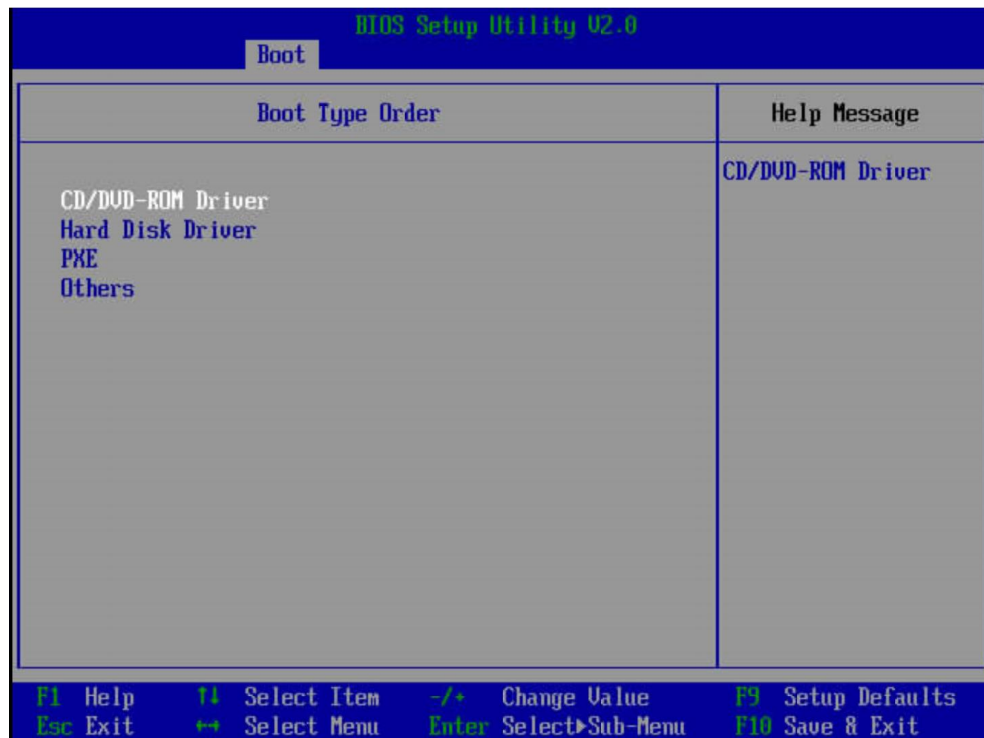
图 6-35 “Boot Type Order”界面
