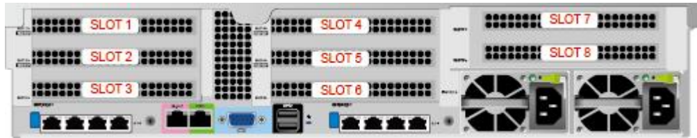
图 3-35 PCIe 插槽
