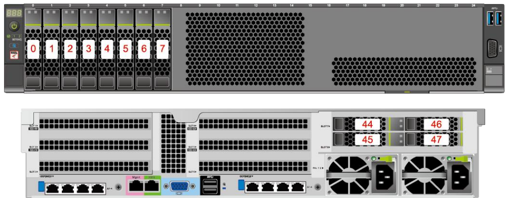
图 3-24 8x2.5 英寸硬盘配置的硬盘编号
