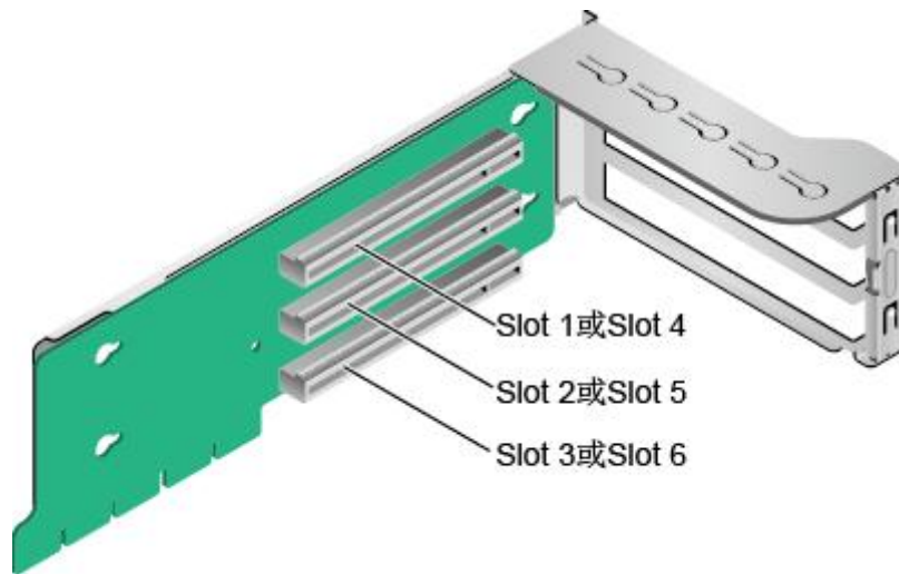
图 3-28 3x8 Riser 卡 1
