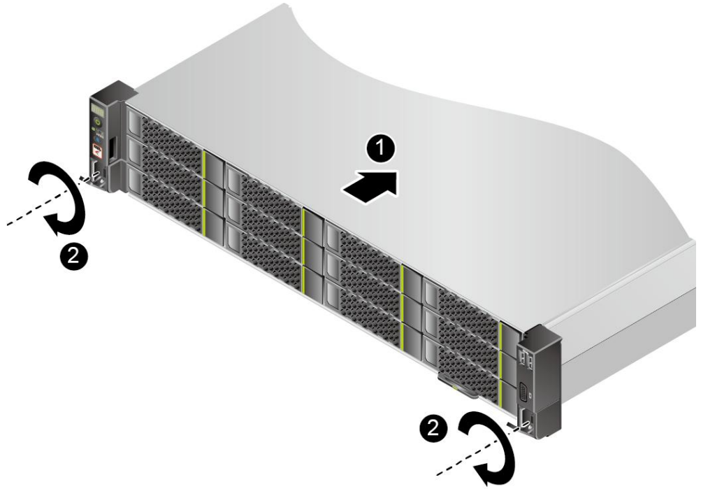
图 6-7 安装服务器
