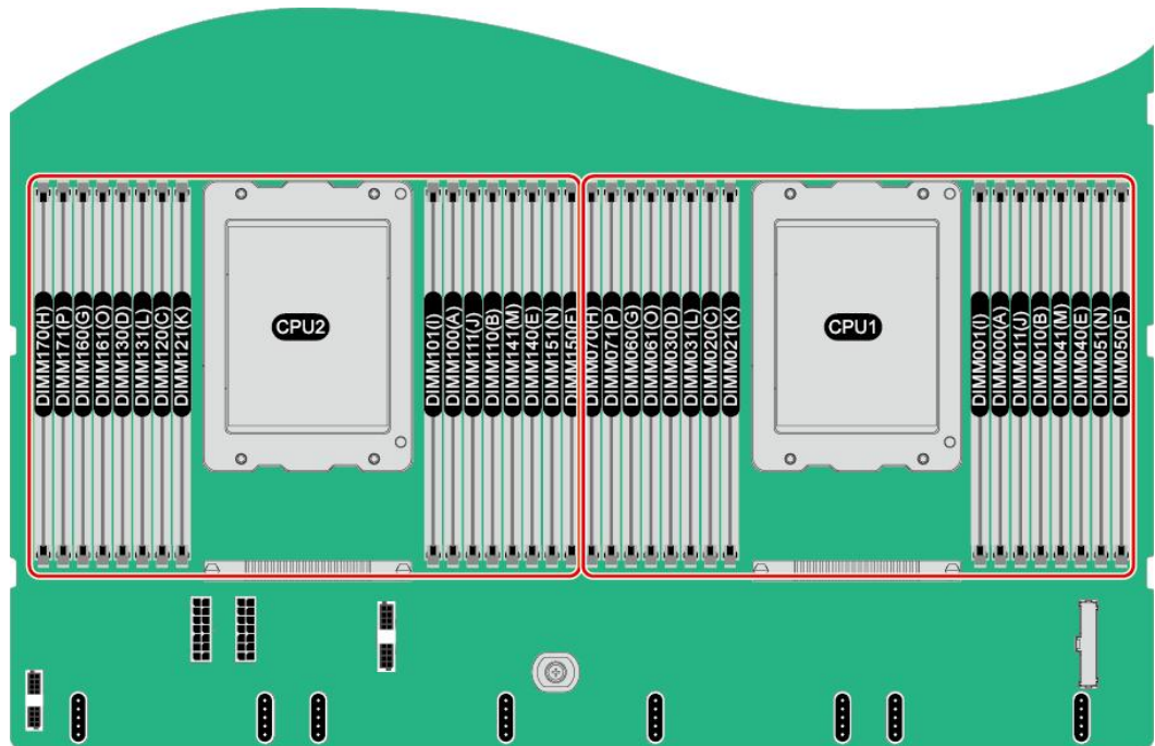
图 3-27 内存槽位编号
